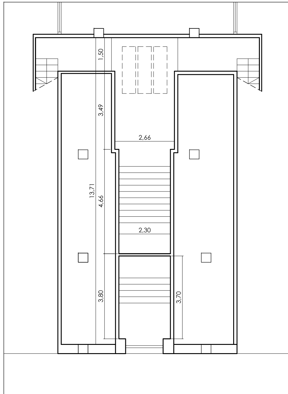
ENTREPLANTA
