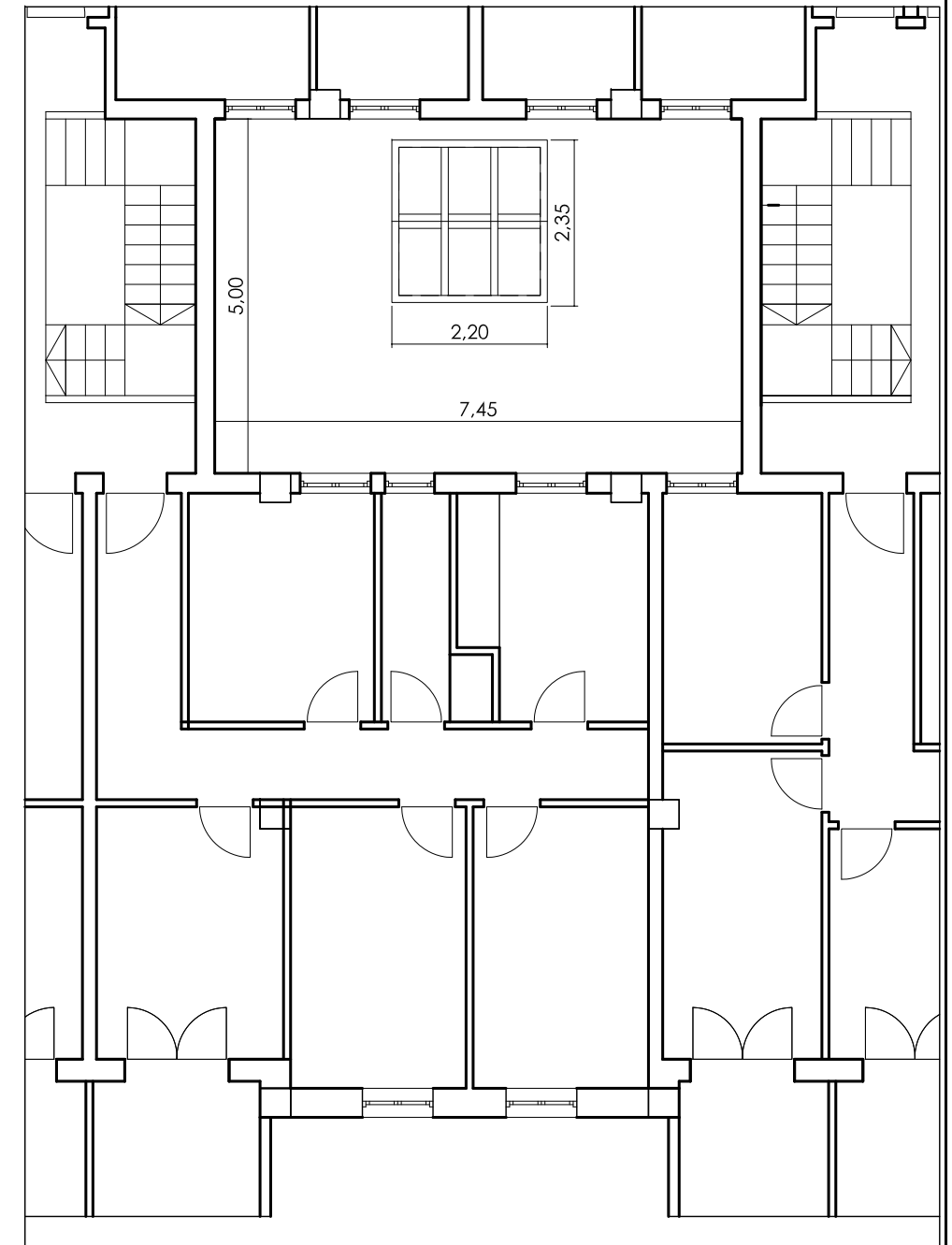
PLANTA PISOS
