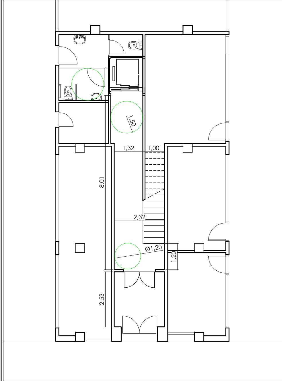
PLANTA BAJA
