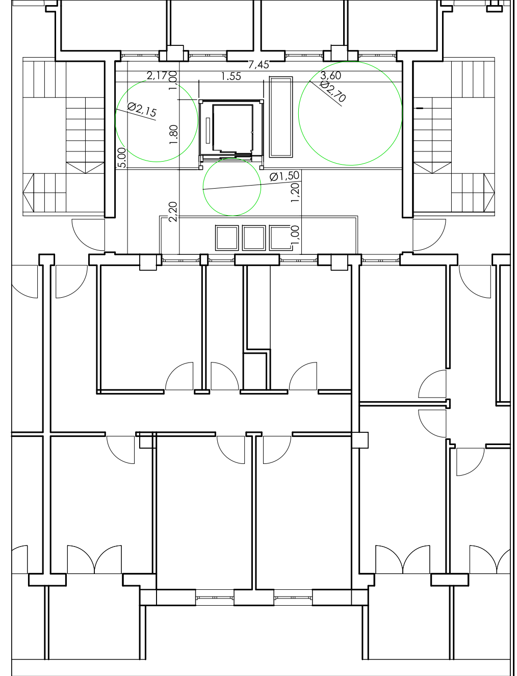
PLANTA PISOS
