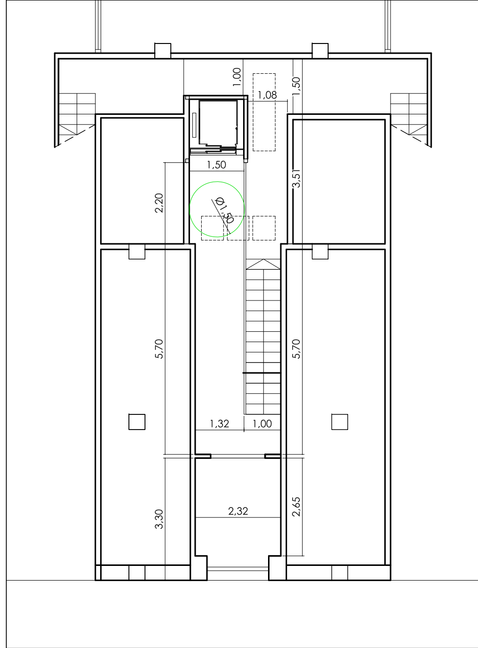
ENTREPLANTA
