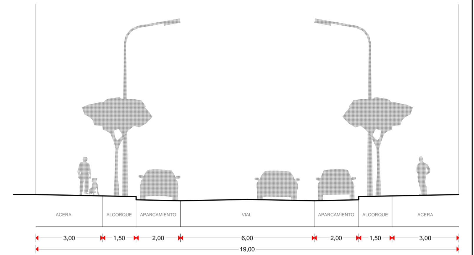
SECCION Calle El Cedro B-B'
