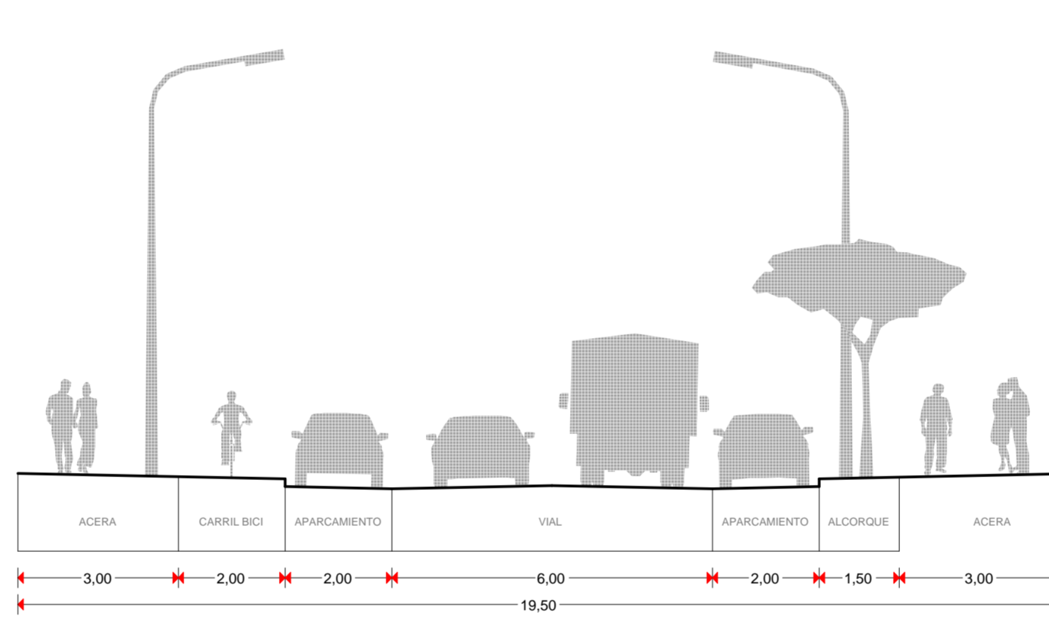
SECCION VIAL Calle El Roble
